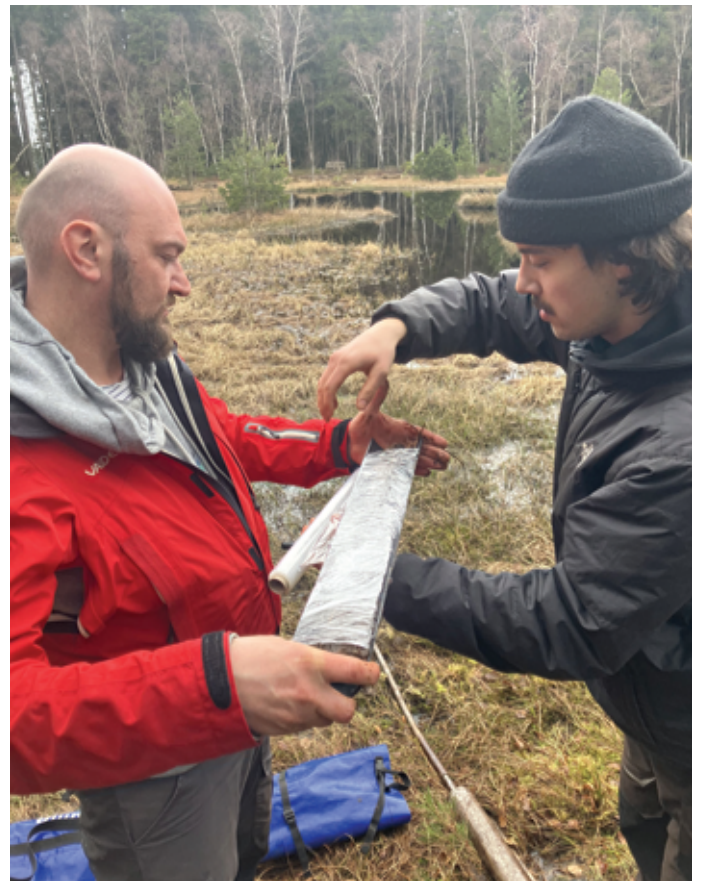
Luftdicht verpackter Bohrkern für den Transport und die Analyse
